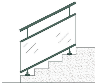
Rampant remplissage verre
