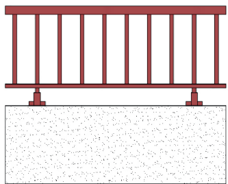
A barreaudage sur muret (hauteur mini du muret 450mm)
