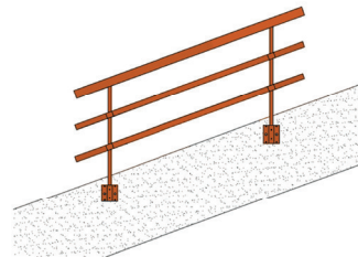
Paquebot avec 2 tubes Ø30 sur muret rampant
