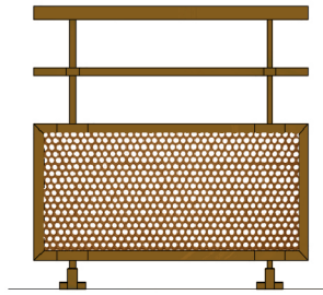
Paquebot à remplissage tôle perforée avec 1 tube Ø30
