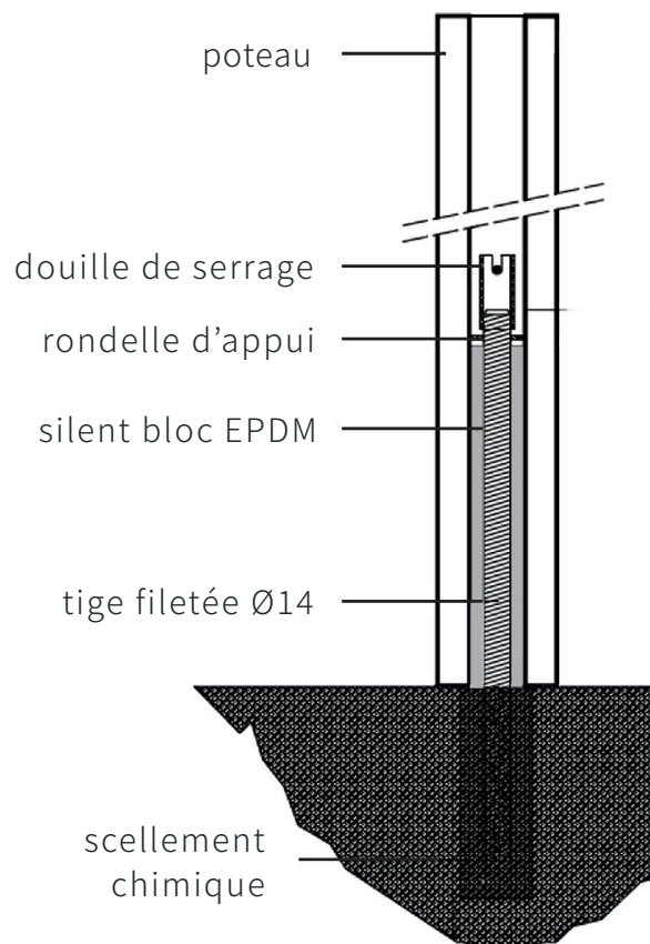
FIXATION DIODON (modèle breveté)
